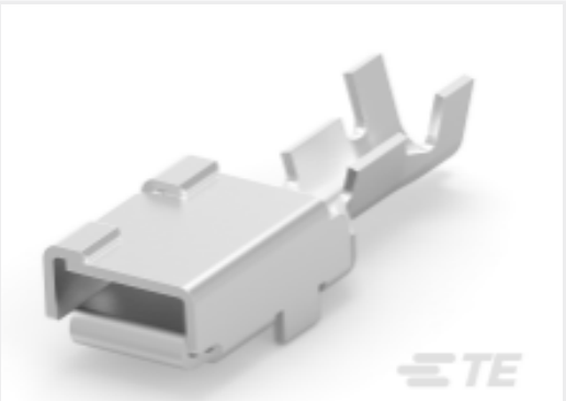
TE 产品编号175038-1 FF 187 REC 0.3-0.5MM2 PTBR
