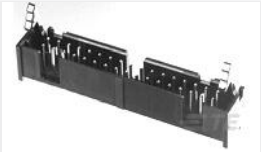
TE 产品编号1-1761608-5 IDC LOW PRO HDR 50P VERT SHT L
