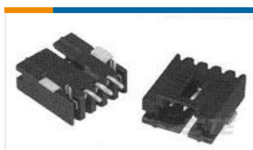
TE 产品编号5-147278-3 04 MTE HDR SRRR SFMNT .100CL
