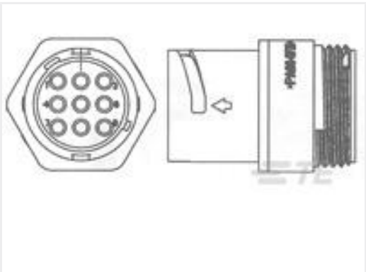
TE 产品编号1445828-3 REC,11-6,FRE HNG,LG INS,STD KE
