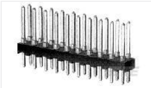
TE 产品编号87227-3 06 MODII HDR DRST UNSHRD .100
