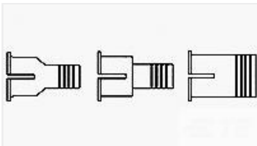
TE 产品编号7-745129-6 SHLDING FERRULE,PLTD,BULK PKG
