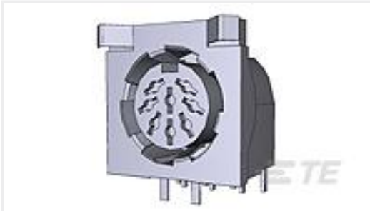
TE 产品编号5787013-1 8 CIRC DIN RCPT W/GRND FINGERS
