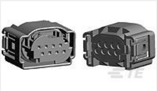
TE 产品编号1-1534229-1 8POS MOS REC COD A
