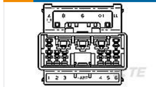
TE 产品编号174942-1 070 MLC W-W CAP HSG 15P
