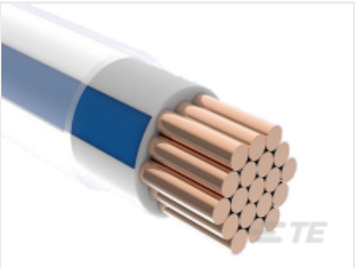
TE 产品编号6131503001 ACW0219-1.00-35(NS)
