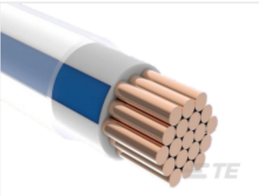
TE 产品编号CT37583001 ACW0219-1.00-30(NS)
