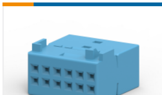
TE 产品编号2278598-1 12POS MQS REC
