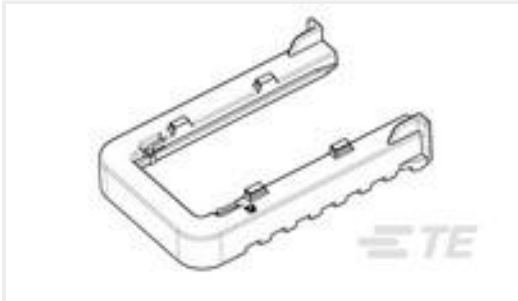
TE 产品编号2112166-2 SLIDE,FOR 21POS.
