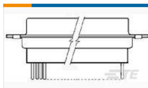
TE 产品编号 208877-1 RECPT ASSY, 104 POSN, AMPLIMITE
