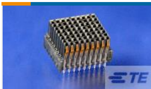
TE 产品编号 1410231-1 MULTIGIG RT T1 1" BP HALF LEFT
