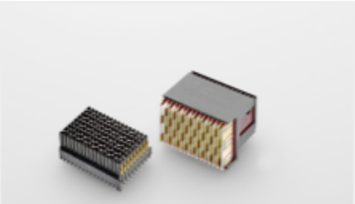
TE 产品编号2302789-1 VERTRECASSY,CENTER,MULTIGIG RT3
