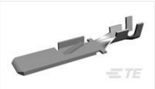
TE 产品编号969031-2 POS-MATE FLA-STE5,2
