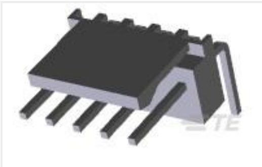
TE 产品编号3-647630-5 05P MTA100 HRD ASSY F/L LF
