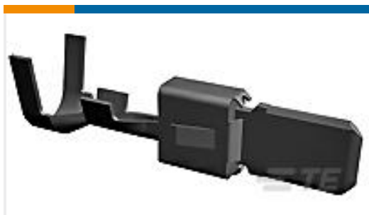
TE 产品编号1-962919-1 TAB 5.8x0.8 CONTACT CS SWS Sn
