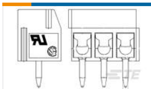
TE 产品编号1776275-4 4P TB ,90deg,VT,3.5mm,Blue,w /interlock
