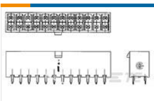
TE 产品编号2-1586037-4 24P VERT HDR VAL-U-LOK V2
