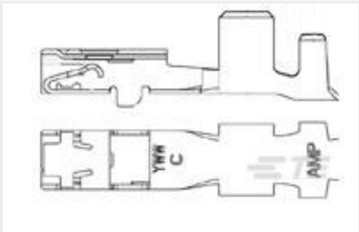
TE 产品编号1326030-2 2.8MM RECP,UNSEAL,18-20AWG
