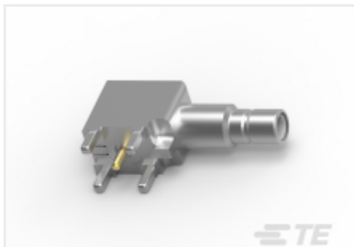
TE 产品编号1274412-1 SMB PCB RIGHT ANGLE JACK
