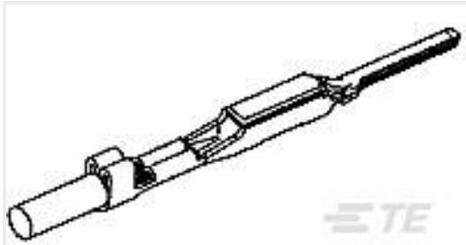
TE 产品编号353537-1 040-3 UNSEALED CONT.TAB(S)
