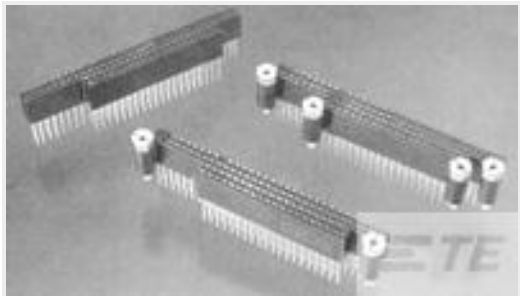
TE 产品编号 1375963-1 PC104 CONN NONSTKTHRU NO STNDO
