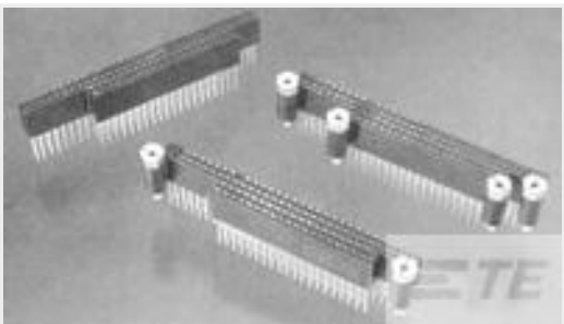
TE 产品编号 1375961-3 PC104 CON NONSTKTHRU 2 STD OF LF
