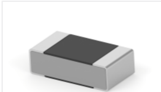
TE 产品编号 6-1879207-2 RN 0603 432K 0.1% 10PPM 5K RL
