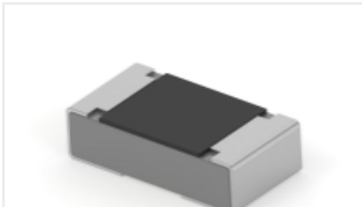
TE 产品编号 5-1879134-1 RN 0603 33K2 0.1% 10PPM 1K RL
