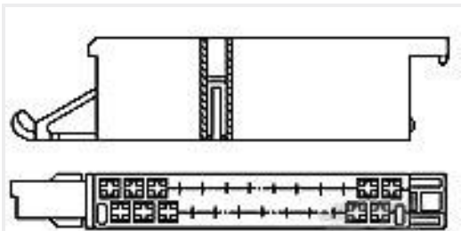
TE 产品编号925470-1 25P MINI TIMER HSG
