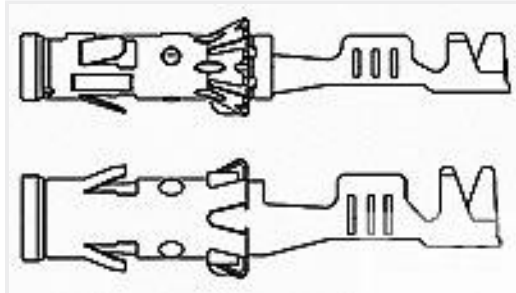
TE 产品编号962956-1 4MM BUCHS-KONTAKT
