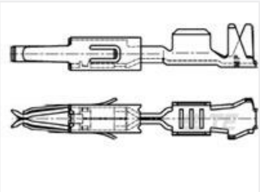
TE 产品编号964263-3 MT2 A REC 1.6 Contact SRC Au
