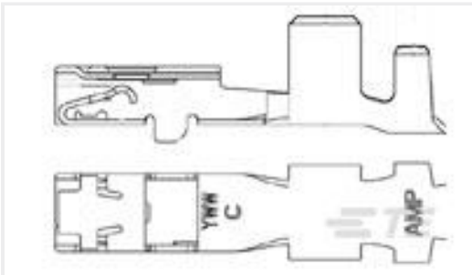
TE 产品编号1326030-7 2.8MM RECP,UNSEAL,14-16AWG,REV
