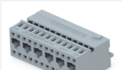
TE 产品编号284225-1 24 POS.RCPT.CONN.HSG.FOR AIRBA
