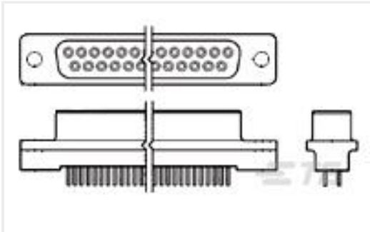
TE 产品编号 745079-4 37 RCPT SP/AP SCRLK
