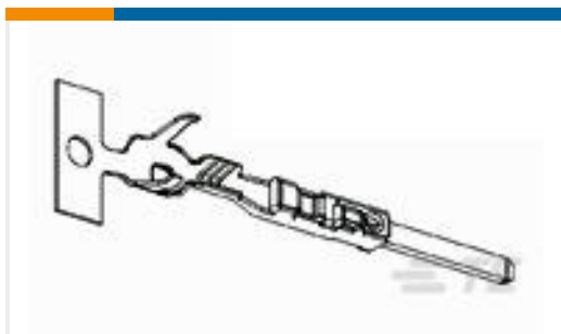
TE 产品编号2141114-3 MCON 1.2 CB TAB SWS AG
