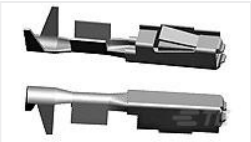
TE 产品编号5-928999-1 MQS0,63 Sn rec LL unseal. >0,2-0,35
