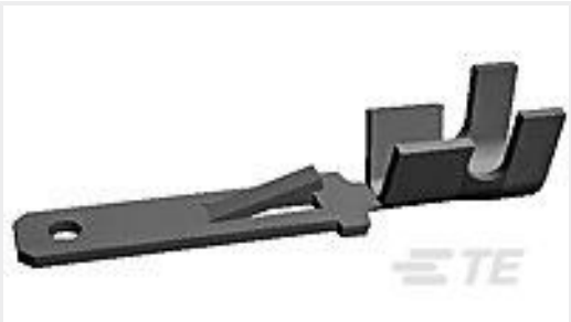
TE 产品编号42098-1 FF 250 TAB 18-14 AWG .032 BR
