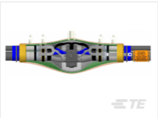
TE 产品编号2832540-1 DDI 240-35(50) v19
