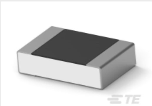
TE 产品编号9-2176376-3 RQ 0805 113K 0.1% 10PPM 1K RL
