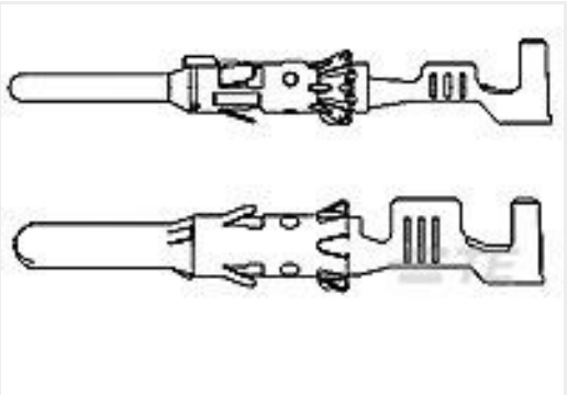
TE 产品编号929964-1 STIFTKONTAKT 2,5MMD
