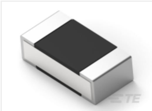
TE 产品编号1-2176307-7 RP 1E 0.1W 18K2 0.1% 25PPM 5K RL
