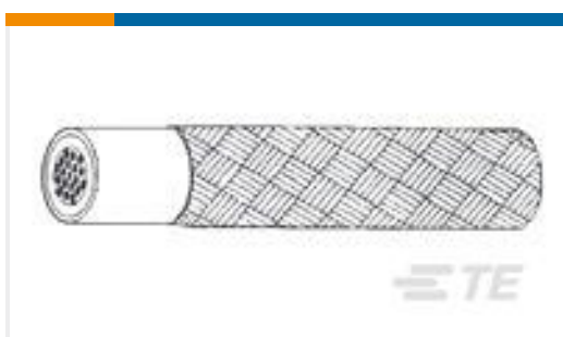
TE 产品编号641671-000 55A3111-20-9
