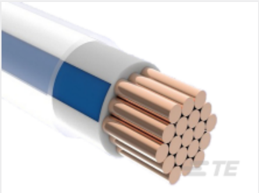
TE 产品编号C519193001 ACW0219-0.75-93(NS)
