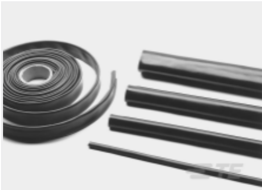
TE 产品编号CAT-R21-T7907237 单壁 RT 770：热缩管，2:1 收缩比
