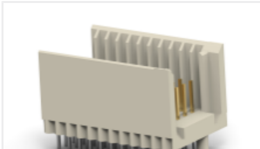
TE 产品编号CAT-472-Z12 硬制公连接器：传统背板，夹层，2mm
