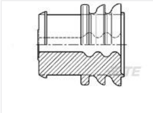
TE 产品编号963244-1 EINZELDRAHTDICHTUNG
