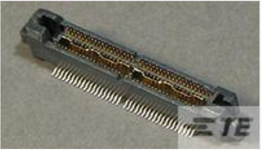
TE 产品编号5767111-9 MICT, PLG, 076, ASY, .025 TAPE CAP
