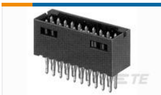
TE 产品编号102699-8 18 MODII HDR DRST SHRD A/PIN
