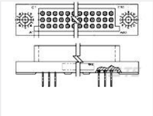
TE 产品编号443857-3 3 ROW BOX RECEPTACLE, 180 POS
