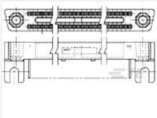
TE 产品编号443851-1 MINI BOX RCPT ASSY/MTG EARS
