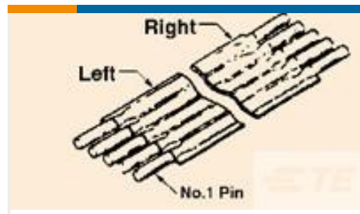
TE 产品编号7-6437138-7 FSN-21.9A-16
