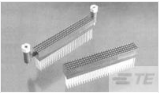
TE 产品编号1375799-4 ASSY, 120 POS PC104 PLUS LF
