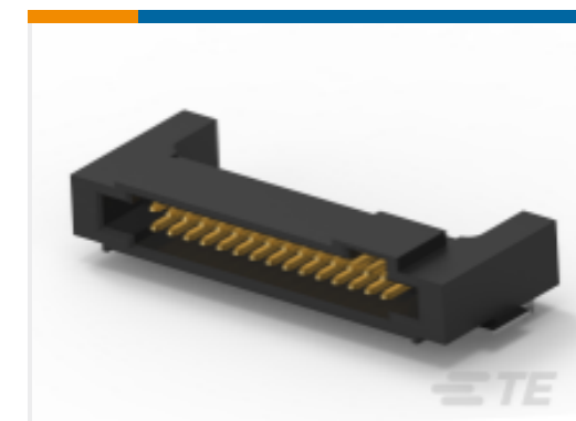
TE 产品编号 104894-7 70 50/50 GRID RA HDR
