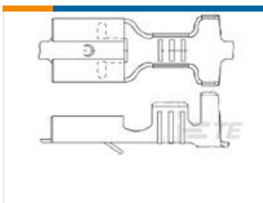
TE 产品编号63833-1 FF 187 REC 18-14AWG BR
